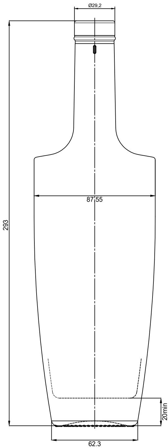
ВИД СПЕРЕДИ
